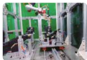
Verschraubung in Leuchteneinheiten
